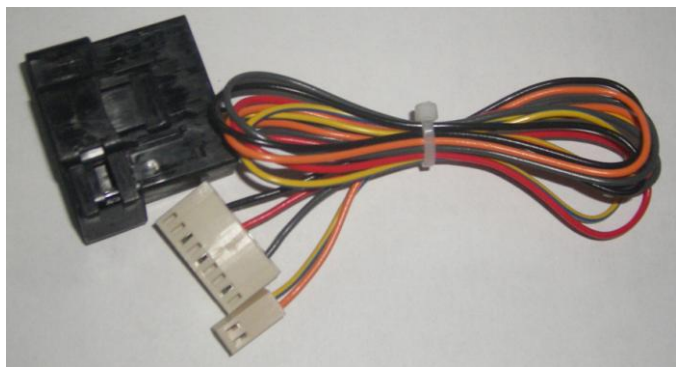
Рис. 1 Жгут для подключения БК
