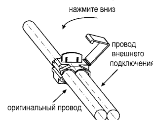
рис.5 Соединение проводов через зажим
