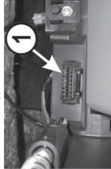
Рис.8 Диагностическая колодка
