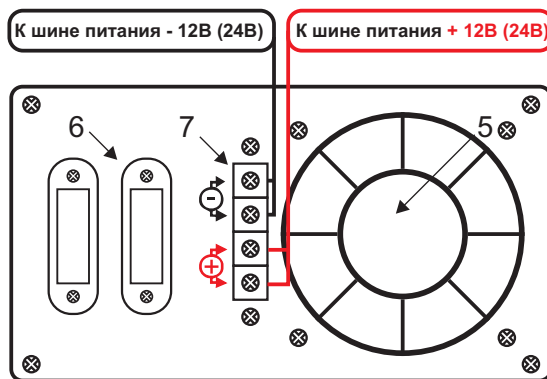
Рис. 2. Задняя панель ПН-92 / ПН-94
